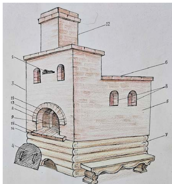
КОНСТРУКЦИЯ РУССКОЙ ПЕЧИ
